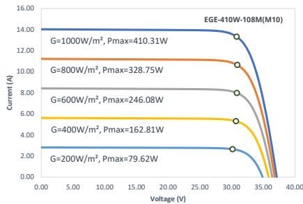
IV-Kurven Bestrahlung
