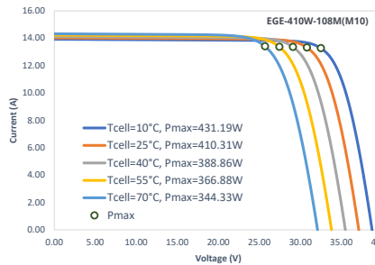
IV-Kurven Temperatur
