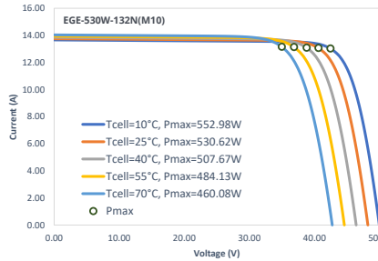
IV-Kurven Temperatur
