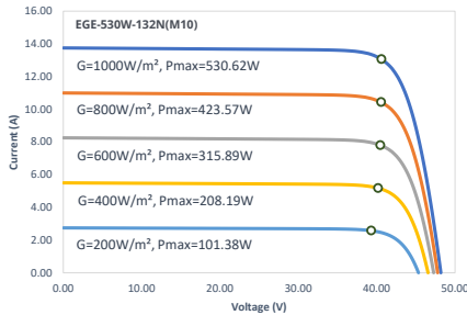
IV-Kurven Bestrahlung
