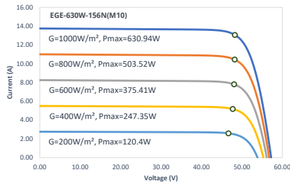
IV-Kurven Bestrahlung
