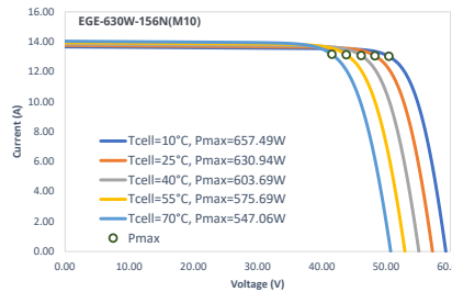
IV-Kurven Temperatur
