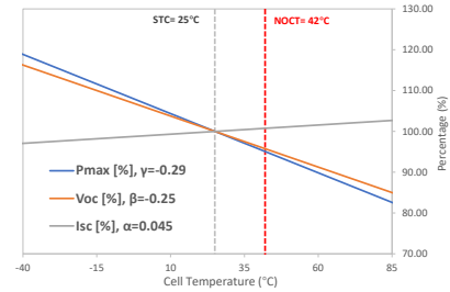
Temperaturabhängigkeit von Isc, Voc, Pmax
