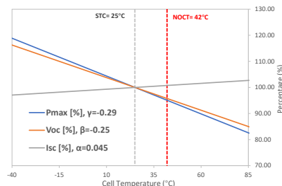
Correlación de temperatura de Isc, Voc, Pmax
