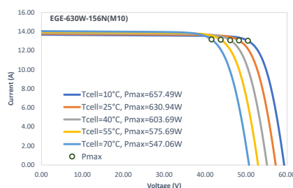
Curvas IV: Temperatura
